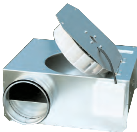
LPKB с загнутыми назад лопатками
