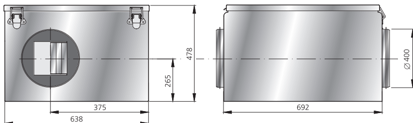
Габариты (mm)
