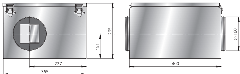
Габариты (mm)
