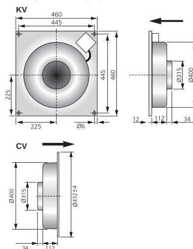
Габариты (mm)
